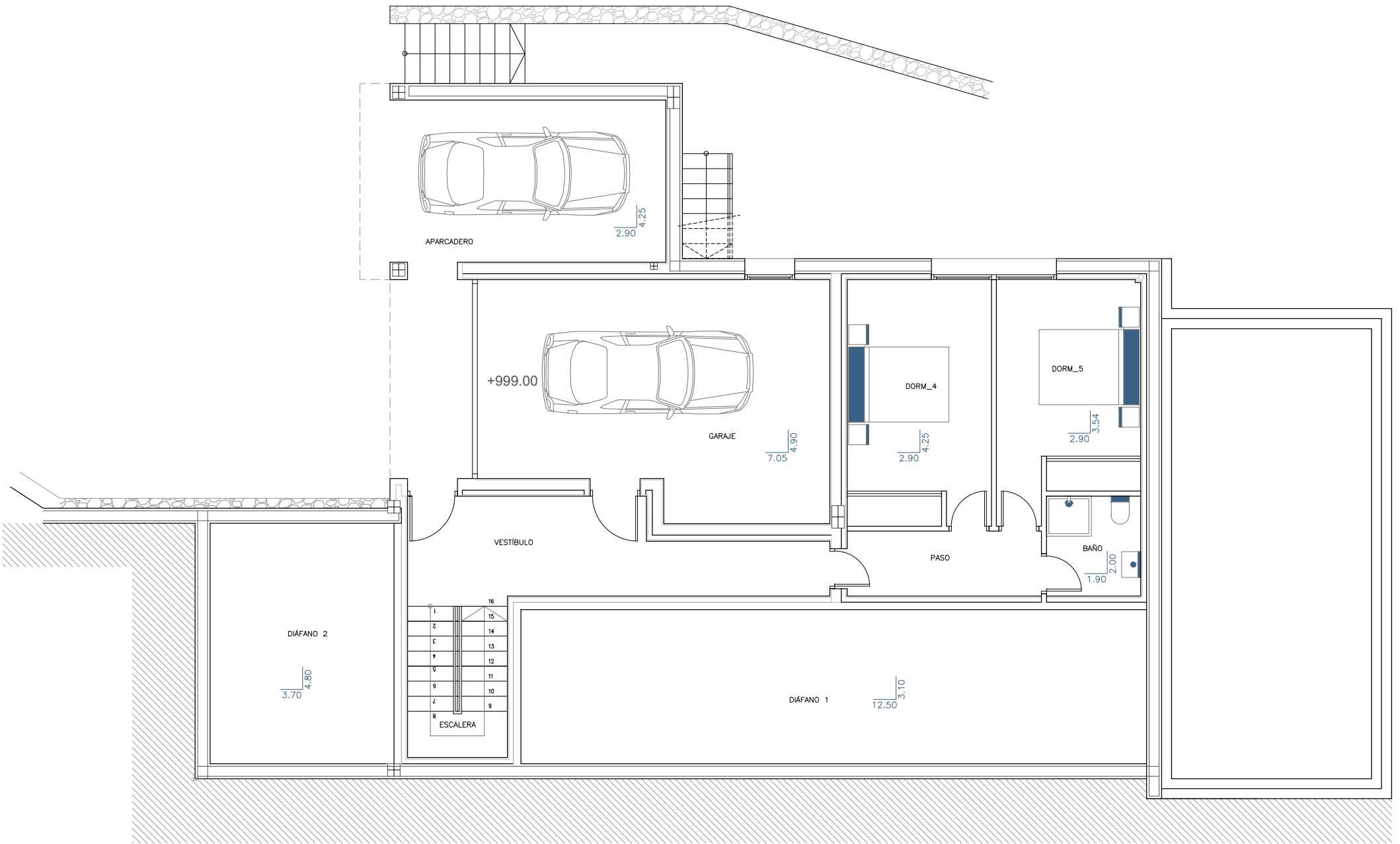
PLANTA SEMISÓTANO
